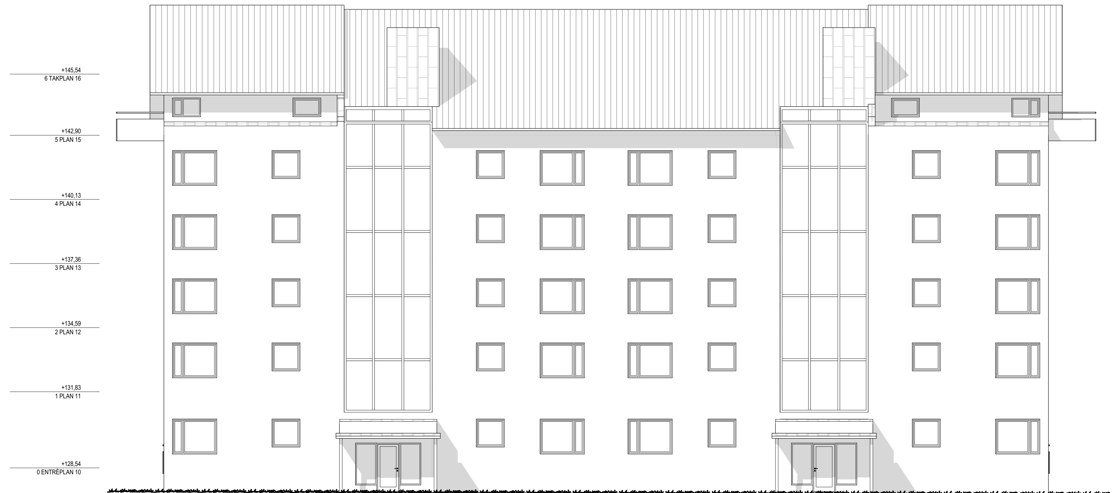
FASAD MOT ÖSTER
