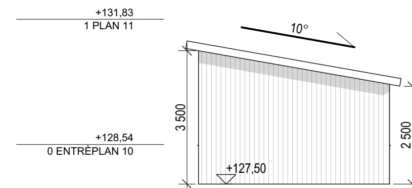
KOPLEMENTBYGGNAD MOT ÖSTER
