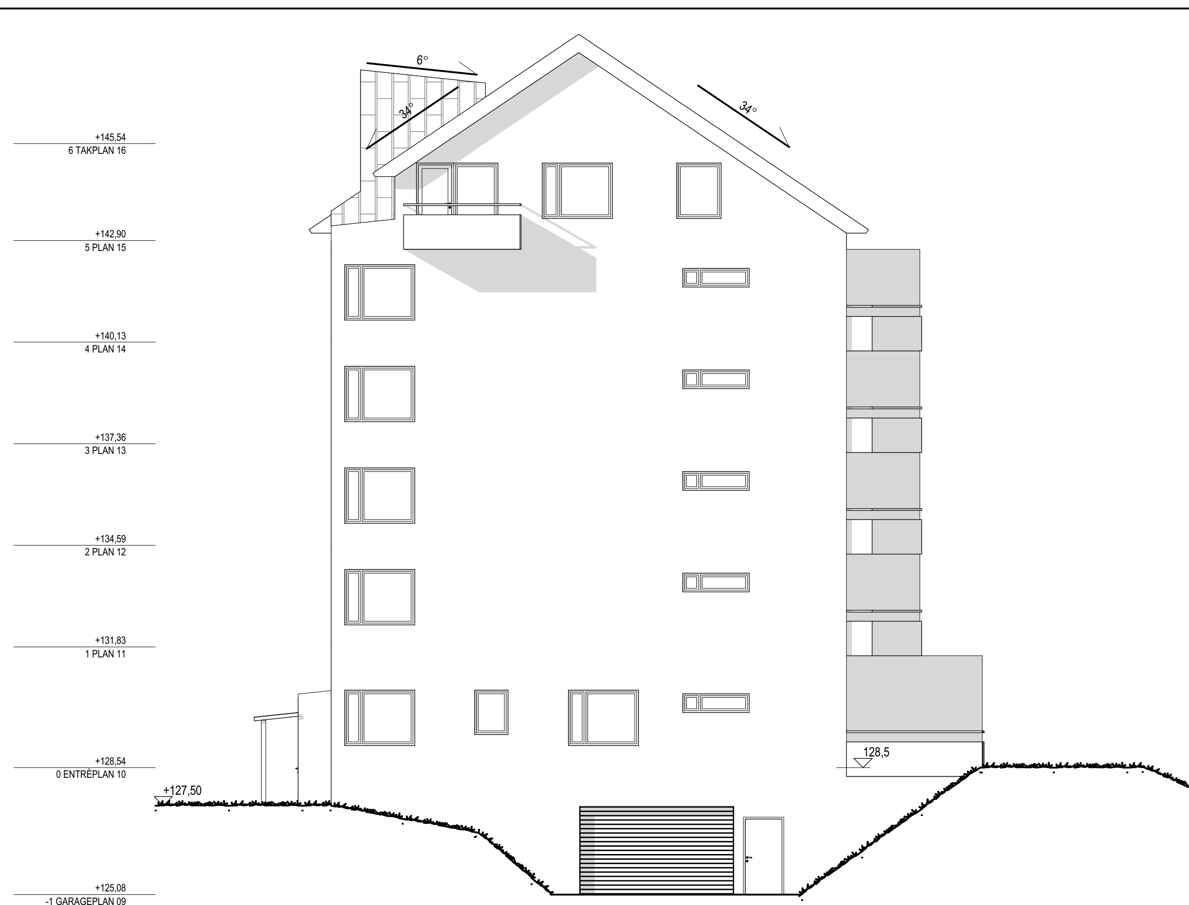
FASAD MOT VÄSTER 1:100
