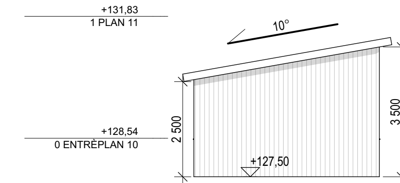
KOPLEMENTBYGGNAD MOT VÄSTER
